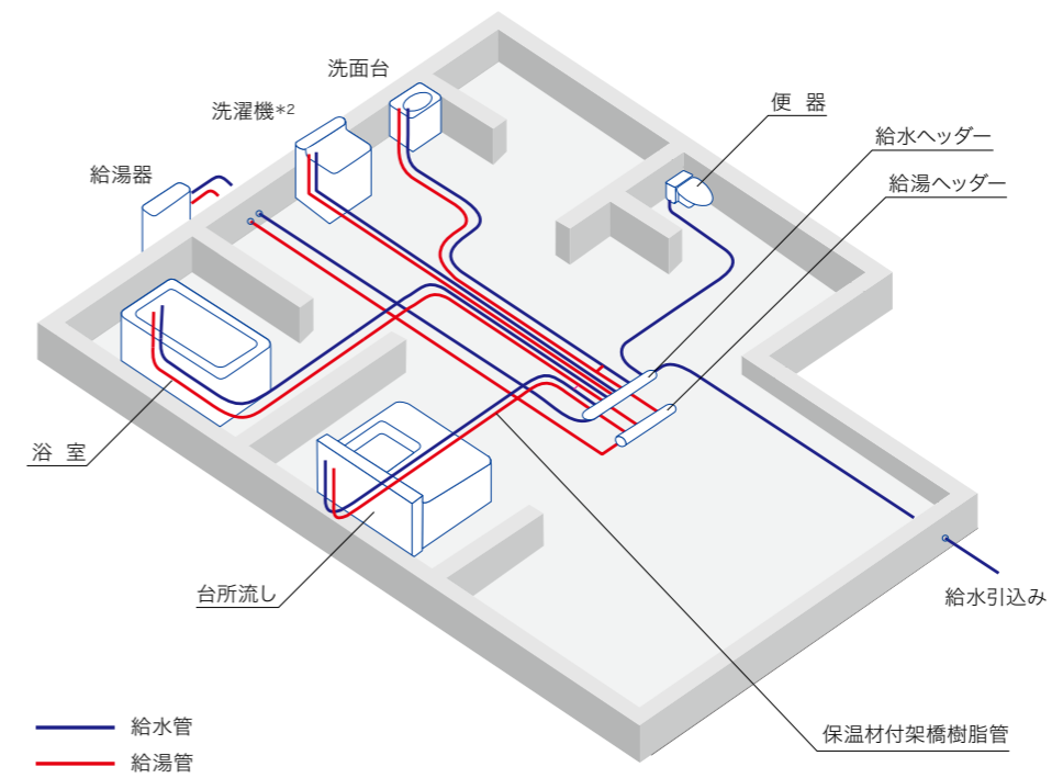
■給水・給湯ヘッダー配管例(概念図)
