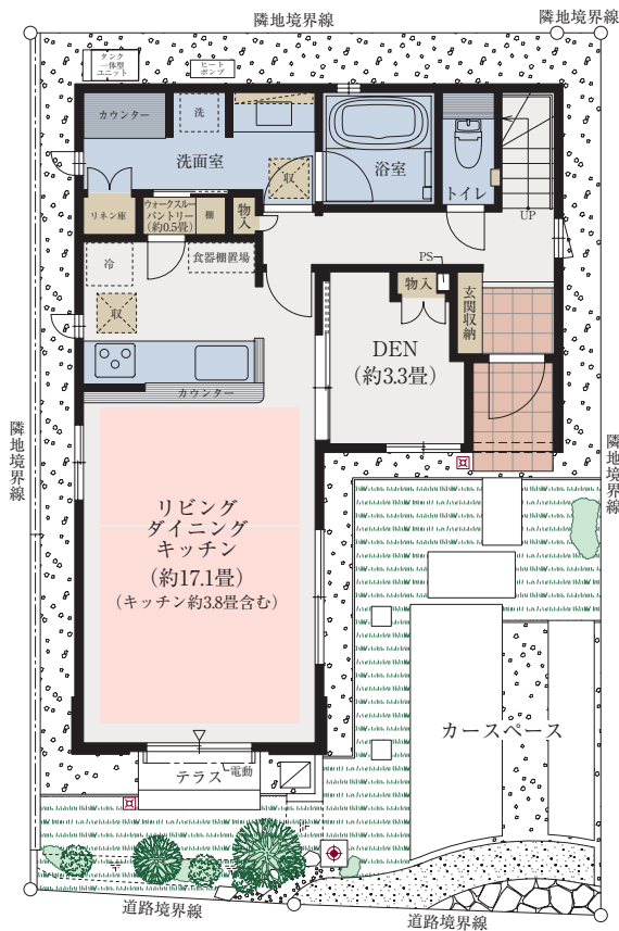
■1階平面図
