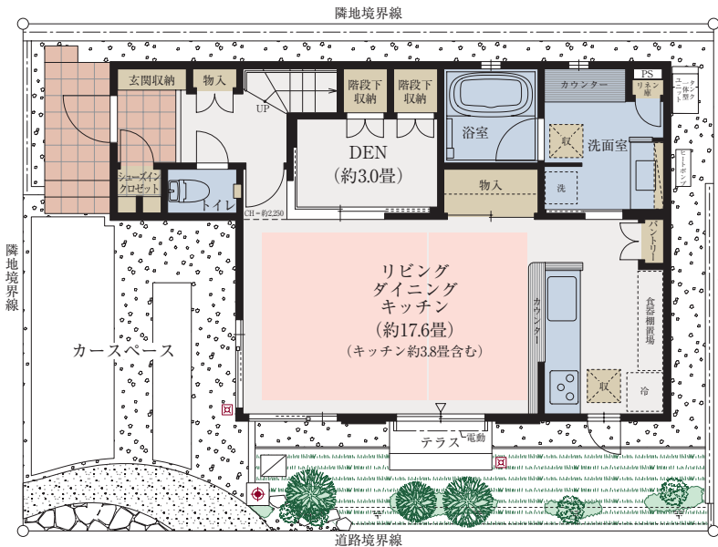
■1階平面図
