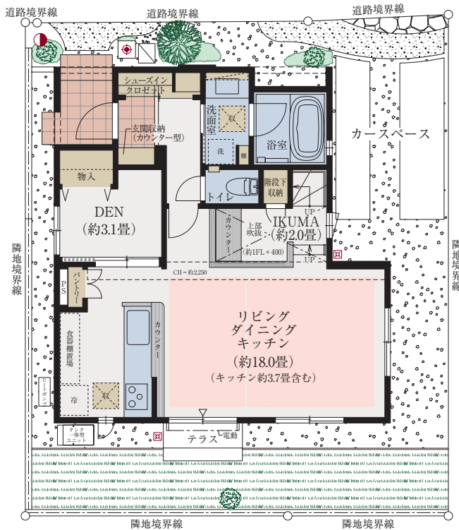
■1階平面図
