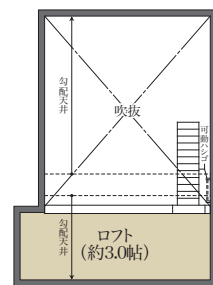
ロフト階平面図
