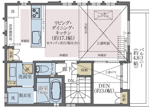
2階平面図
