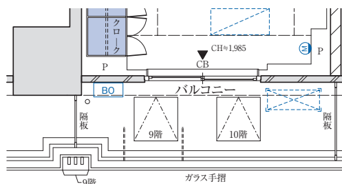
●9・10階部分図
