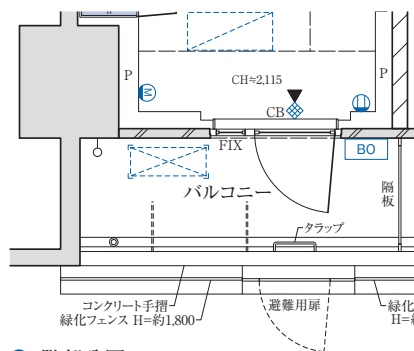
●1階部分図
