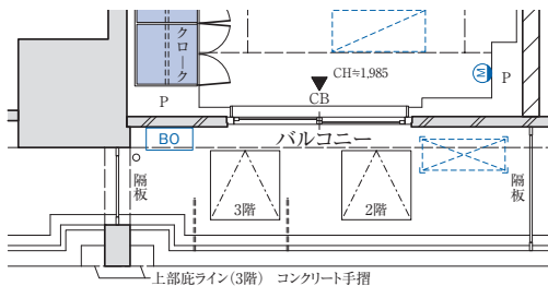
●2・3階部分図
