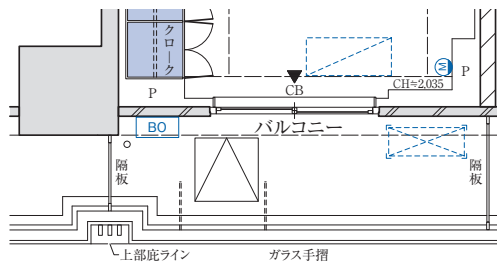
●11階部分図
