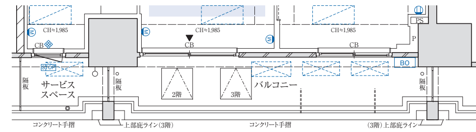
●2・3階部分図
