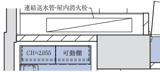
●11階部分図
