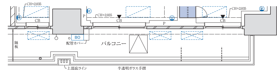
●11階部分図
