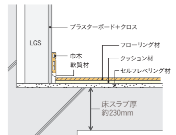
直床(参考写真) *メーカーにより仕様異なります。 *洗面室・一部トイレは二重床となります。
