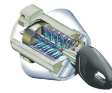
ディンプルシリンダー概念図
