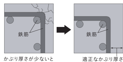
かぶり厚さ概念図
