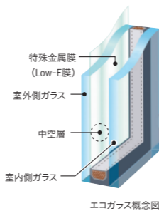
エコガラス概念図
